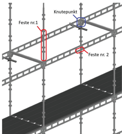
Figur 1.2 Anbefalte festepunkter
